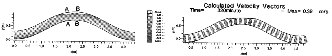
図-7 蛇行部計算結果(2)(水制を死水域化)
