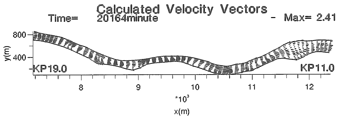
図-12 札内川計算結果(流速ベクトル図)
