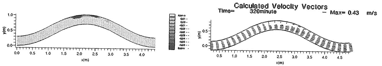
図-5 蛇行部実験結果
