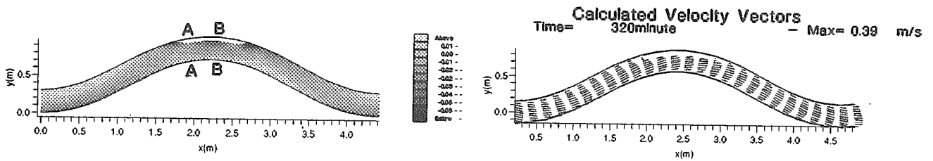
図-6 蛇行部計算結果(1)(水制を粗度化)
