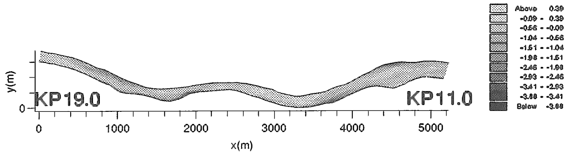
図-9 横断形状変化比較
