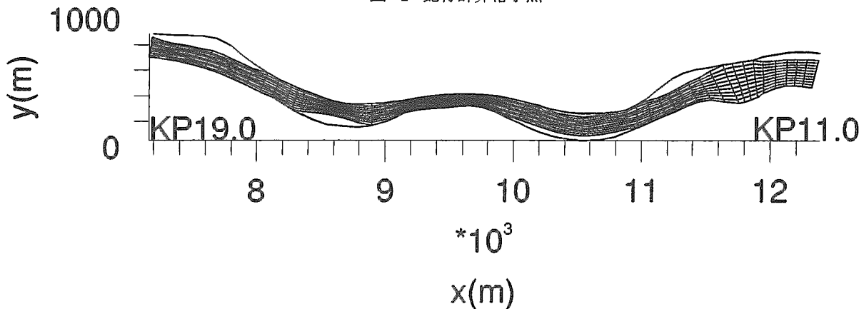
図-1 蛇行計算格子点
