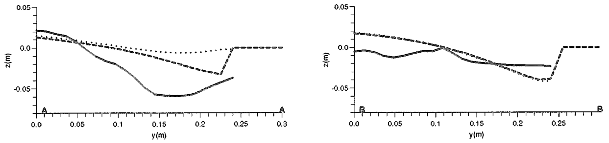
図-9 横断形状変化比較
